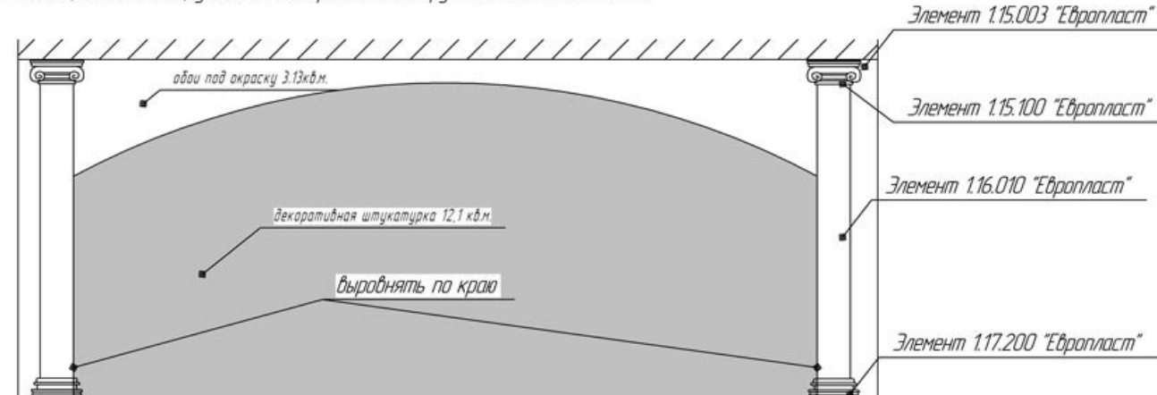
Размещение лепнины, указание материалов конструктивного элемента №3
