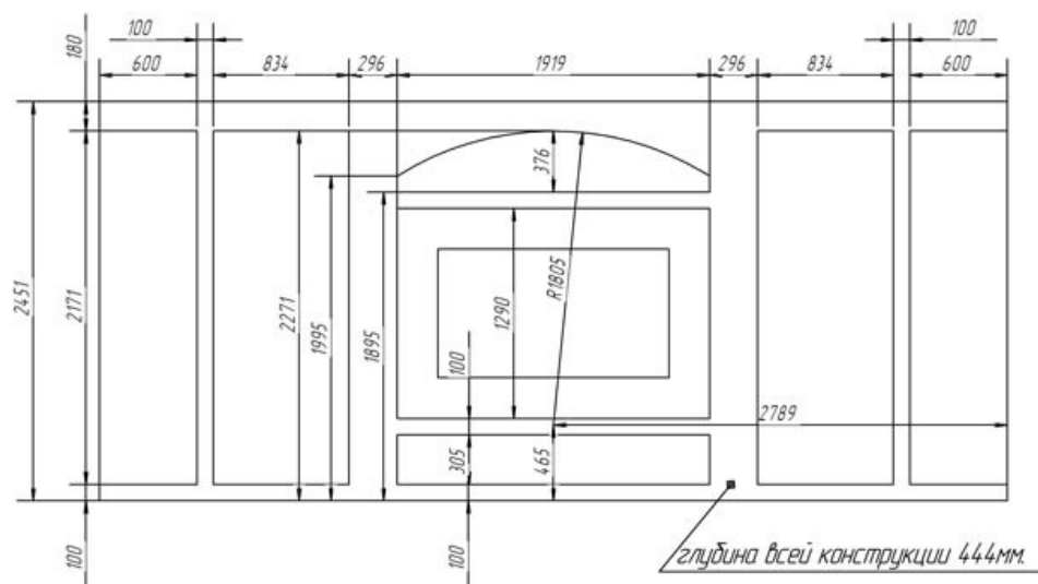
Построение конструктивного элемента №1
