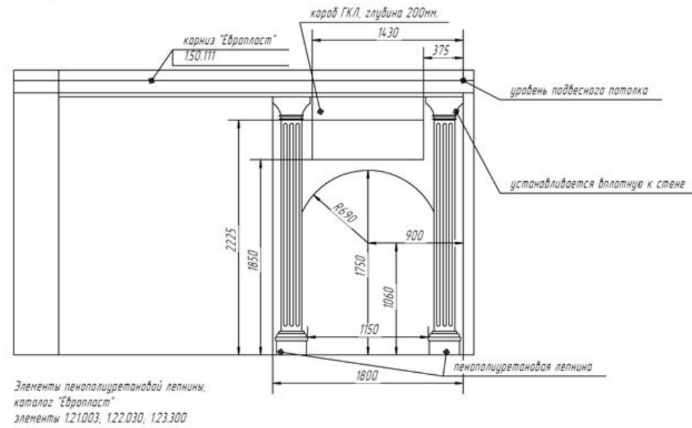
Конструктивный узел №1
