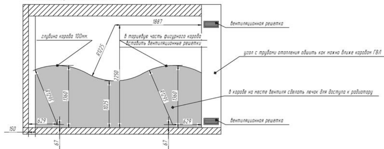
Построение конструктивного элемента №1
