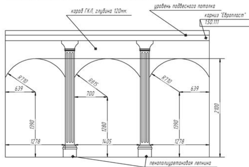
Конструктивный узел №3
