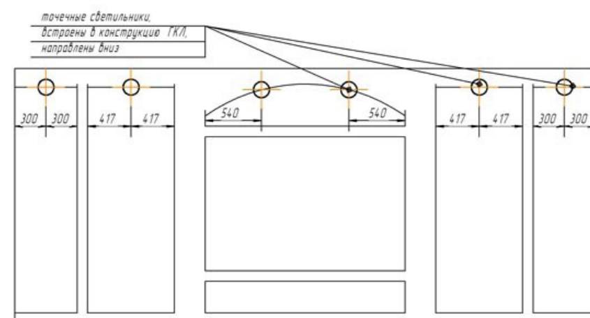
Размещение освещения конструктивного элемента №1
