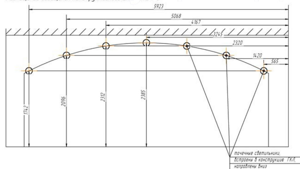
Размещение освещения конструктивного элемента 13
