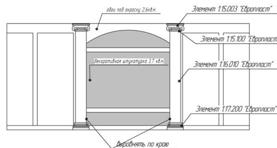
Размещение лепнины, указание материалов конструктивного элемента №1
