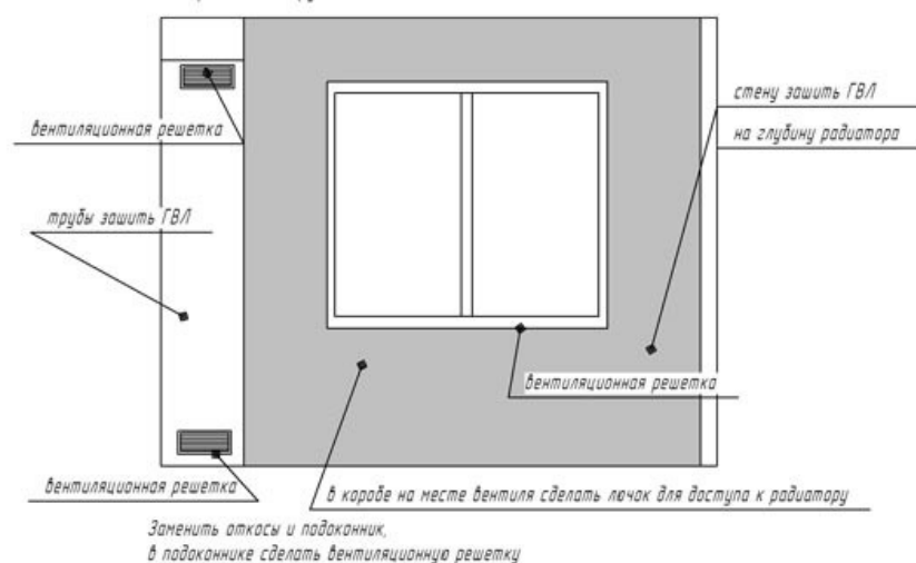
Построение конструктивного элемента №2
