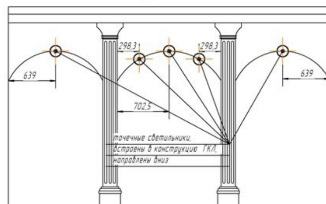
Конструктивный узел №3
