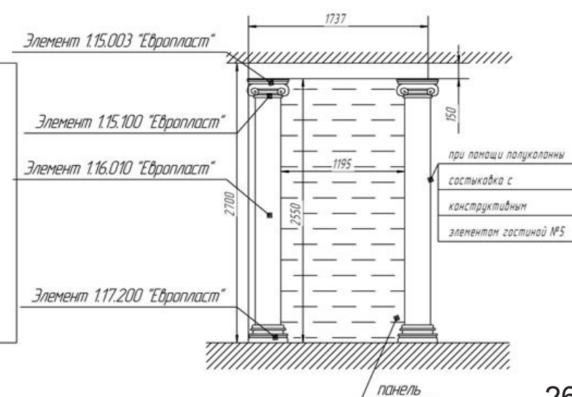
Аква-панель
