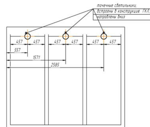
Размещение освещения конструктивного элемента №4
