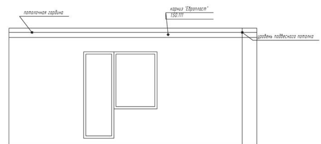
Конструктивный узел №4
