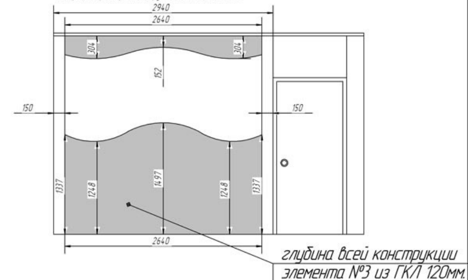
Конструктивный узел №3
