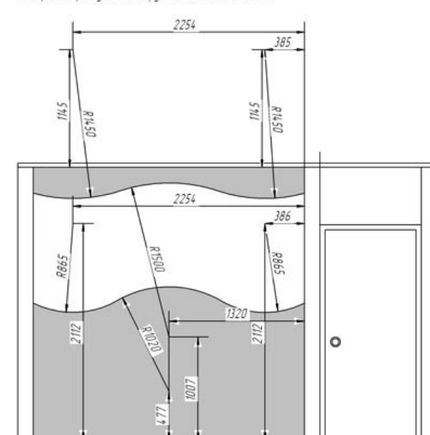
Построение радиусов конструктивного элемента №3
