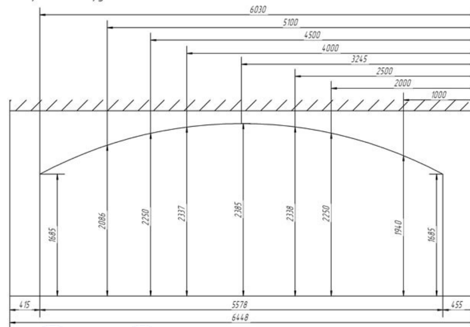
Построение конструктивного элемента №3
